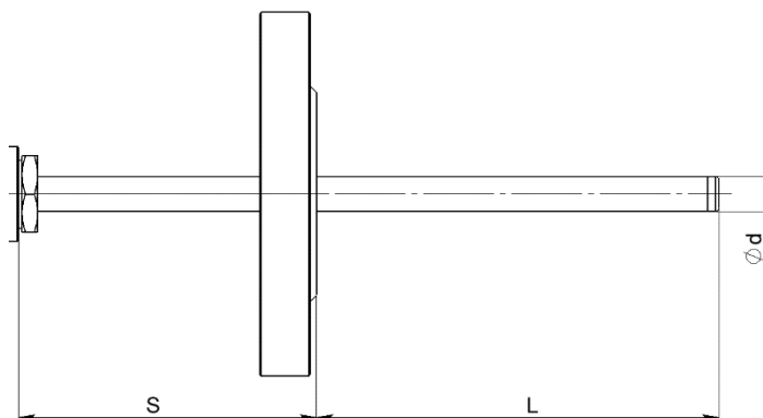
Рисунок А.5 – Термопреобразователи модификаций CTR, CTU с вынесением монтажной головки
