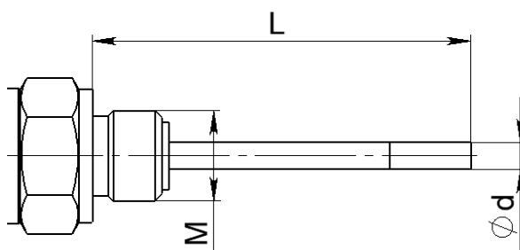
Рисунок А.3 – Термопреобразователи модификаций CTR, STU без вынесения монтажной головки
