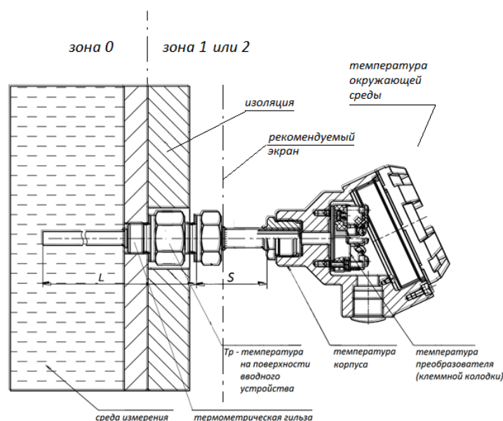
Рисунок 2 – Определение температуры первичного преобразователя или термопреобразователя
